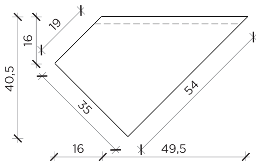
PIANTA | PLAN
