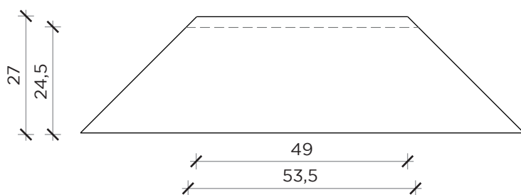
PIANTA | PLAN
