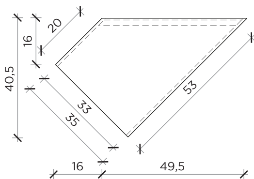
PIANTA | PLAN
