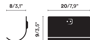
Dettaglio della mensola / Detail of the shelf
