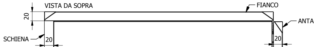
VISTA DA SOPRA
