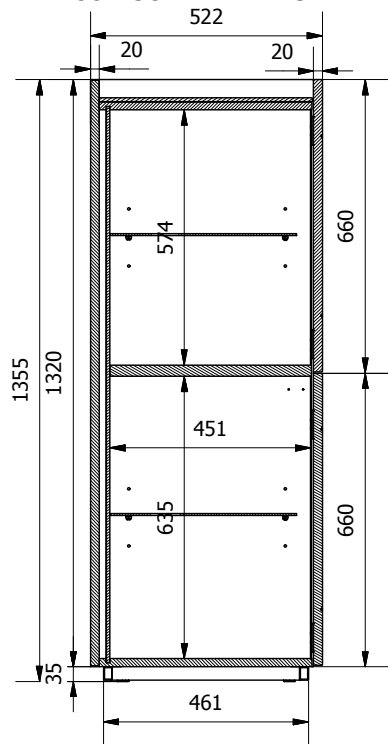
SEZIONE VANO ANTA MADIE 15.66 CON SCHIENA A VISTA
