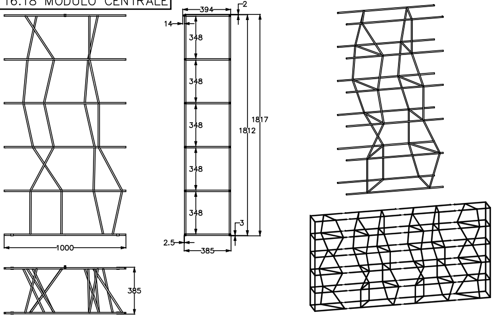
Art. 16.18 MODULO CENTRALE
