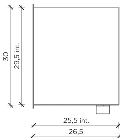
LATO | SIDE
