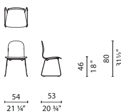
TW_3 / TW_30
