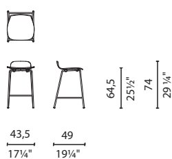
TW_11B / TW_11BO
